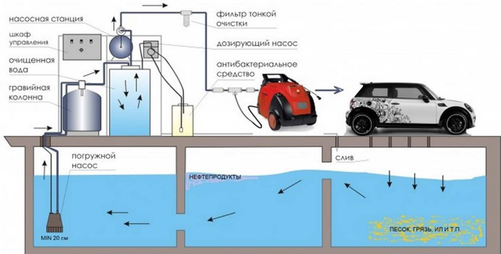
Схема размещения оборудования на автомойке
